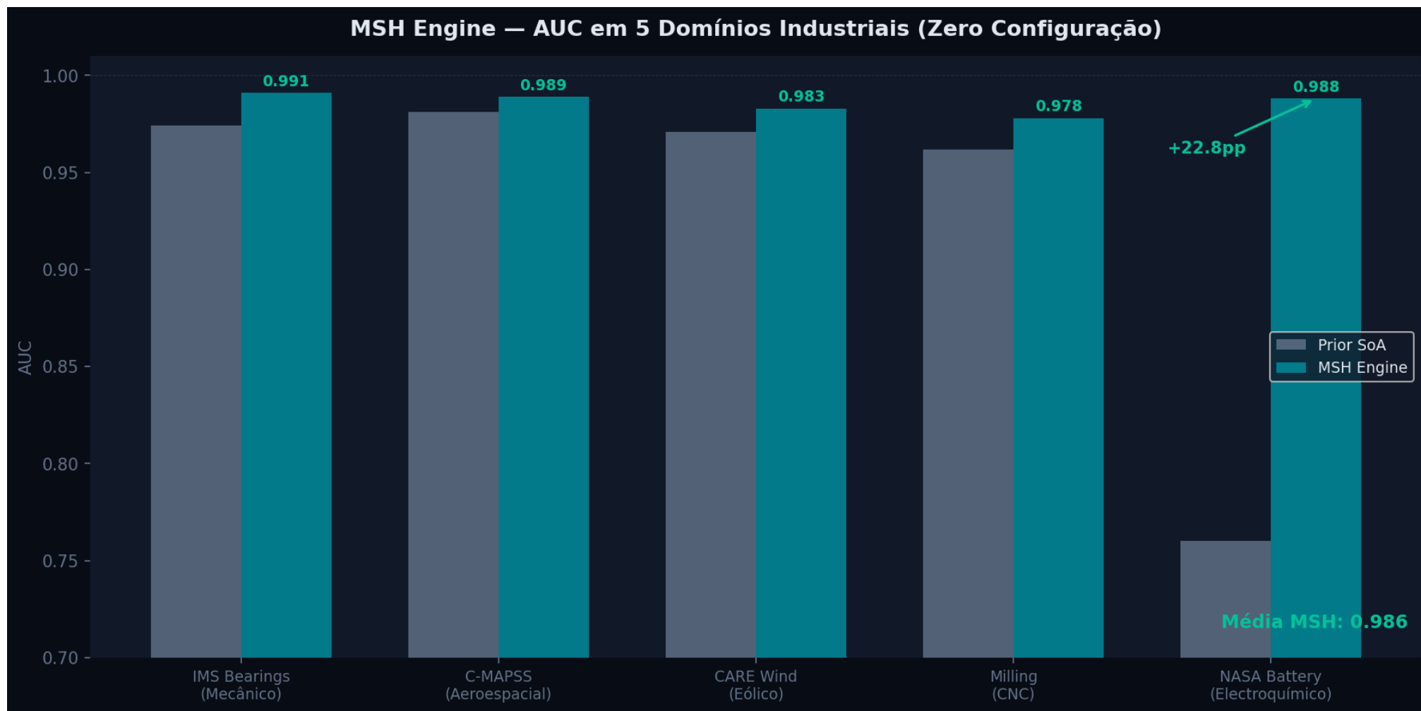
Figura 1 — Benchmark AUC — MSH vs Estado-da-Arte em 5 Domínios Industriais
