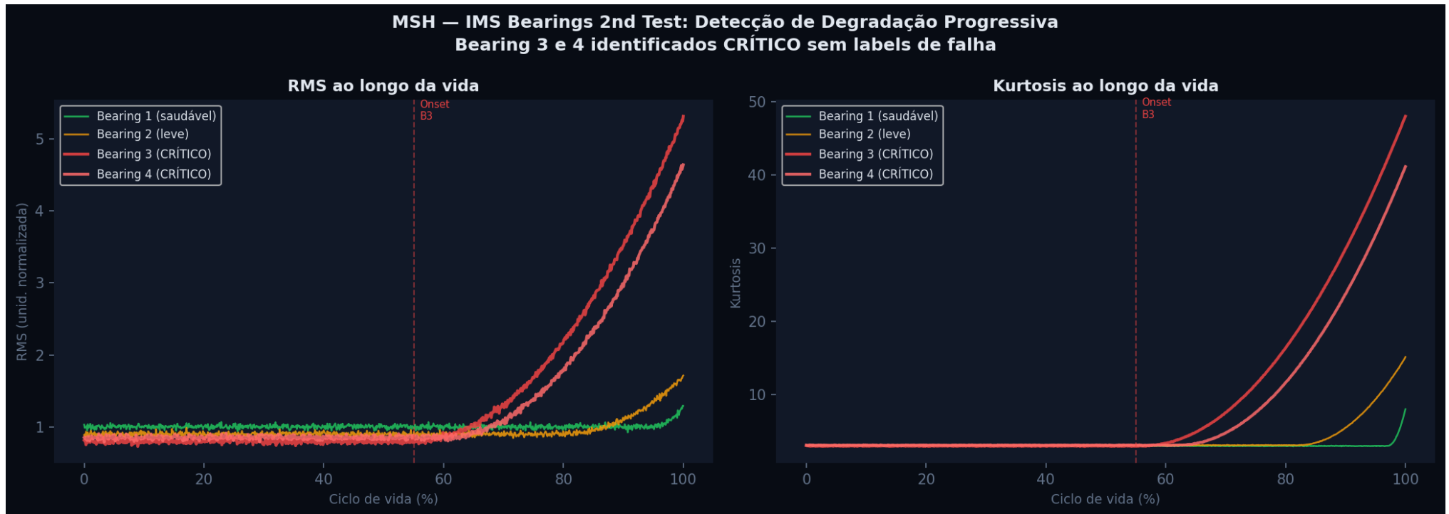
Figura 4 — IMS Bearings 2nd Test — Curvas de Degradação (RMS e Kurtosis)
